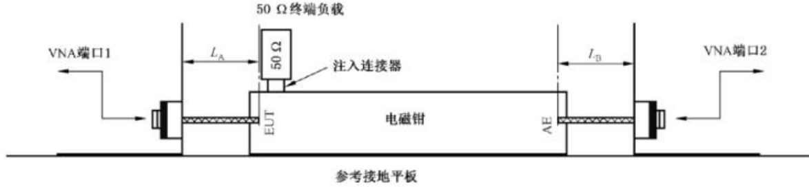
图 A.6 阻抗/去耦系数测量布置
