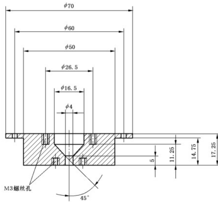
c) 剖面图
