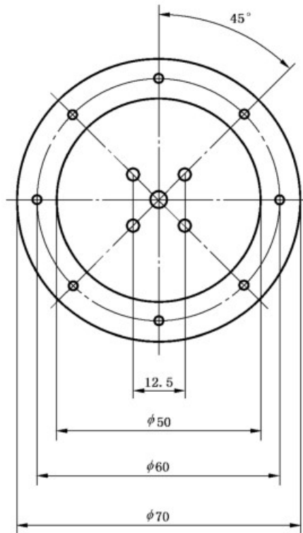
b) 仰视图
