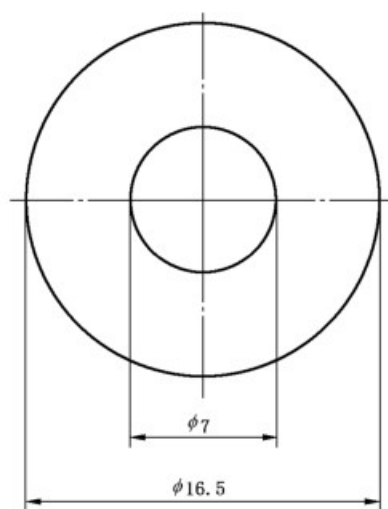
d) PTFE 部件 II 俯视图
