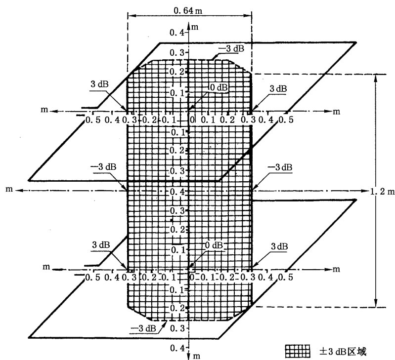
图 B.5 两个相距 0.8 m 的(边长为 1 m)正方形感应线圈在中央垂直平面上产生的磁场的 3 dB 区域(垂直于线圈平面的分量)示意图
